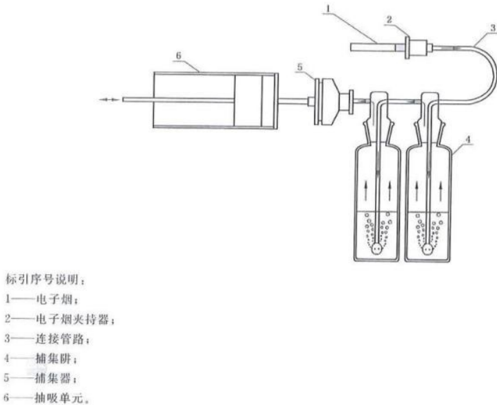
图 F.2 电子烟抽吸连接方式示意图
